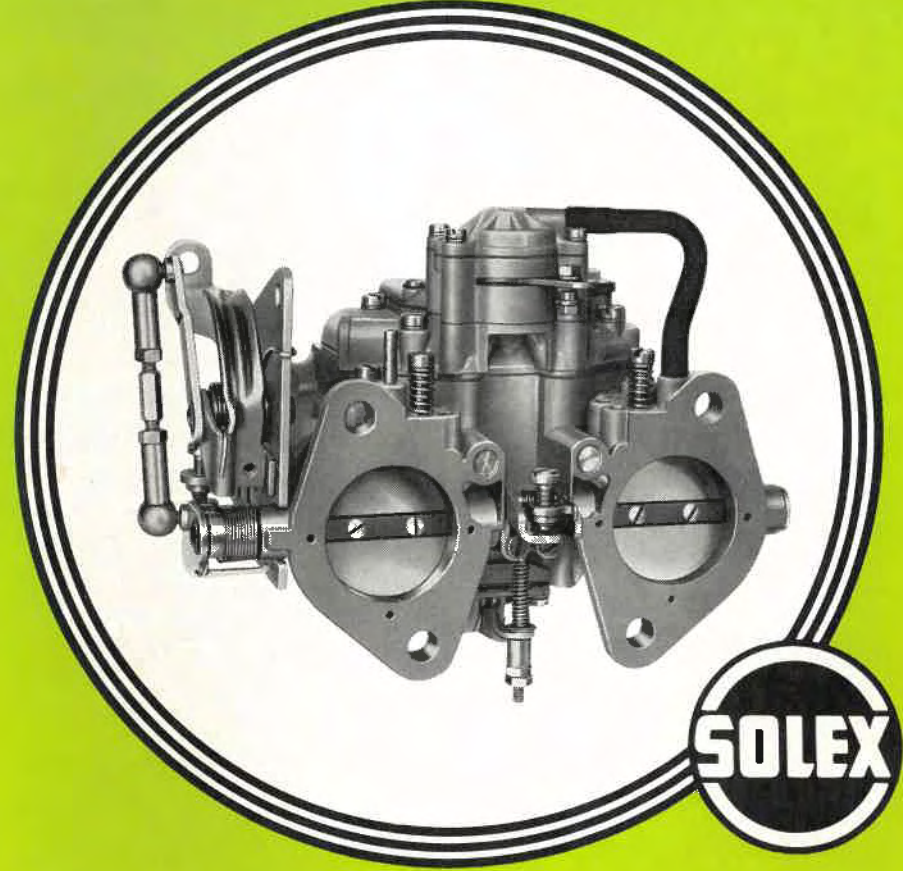
Doppel-Fallstromvergaser 40 DDH
