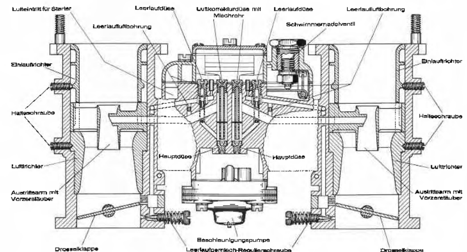
Bild 12: Doppel-Fallstromvergaser 40 DHH (schem. Schnitt)
