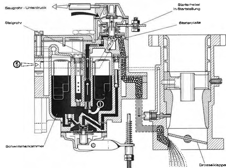
Bild 6: Wirkungsweise beim Kaltstart
